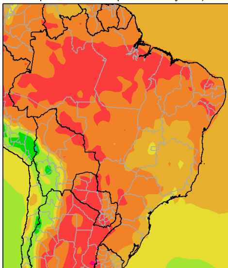
Perspectiva Climática del 12 al 18 de Diciembre 2013 Temperatura Maxima (Grados Centigrados)
